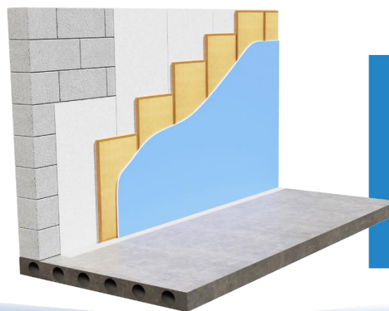
ШУМОИЗОЛЯЦИЯ СТЕН И ПЕРЕГОРОДОК. БЕСКАРКАСНАЯ БАЗОВАЯ СХЕМА
